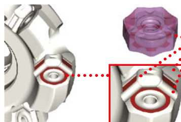
Powierzchnie styku
